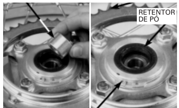
ANEL ELÁSTICO/ARRUELA
