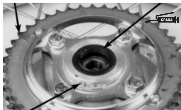
ANEL ELÁSTICO/ARRUELA
