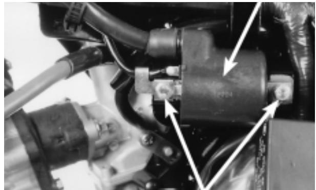
PARAFUSOS MÓDULO DE CONTROLE DA IGNIÇÃO
