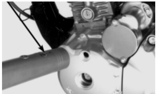
TAMPA DO ORIFÍCIO DE SINCRONIZAÇÃO LUZ ESTROBOSCÓPICA
