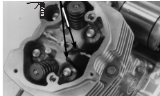
CABEÇOTE PARAFUSO/ARRUELA DE VEDAÇÃO HASTES DE ACIONAMENTO
