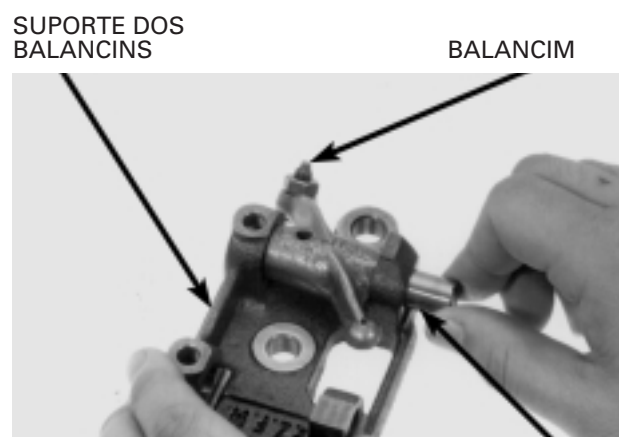
EIXO DO BALANCIM
