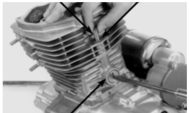
EIXO DOS BRAÇOS OSCILANTES
